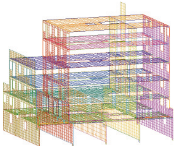
Bild 5. FEM-Gebäudemodell (Längswände ausgeblendet) Fig. 5. FEM-Model (longitudinal walls hidden)
