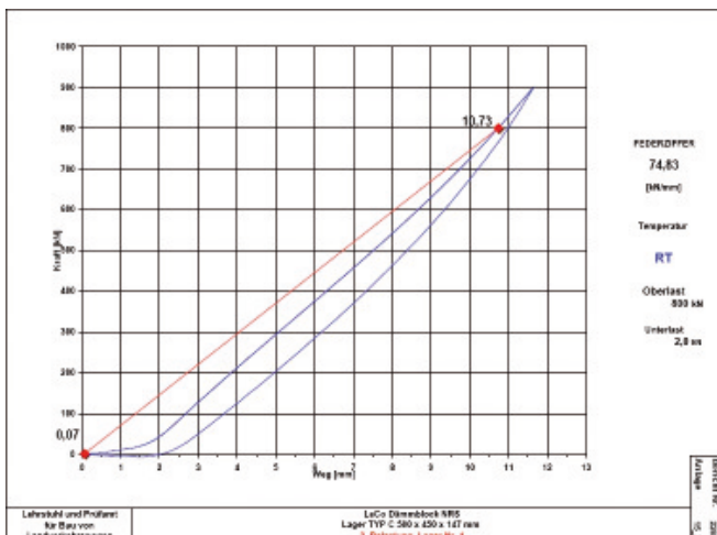
Bild 10. Kraft-Verformungs-Diagramm (Typ C) Fig. 10. Force-deformation-diagram (type C)
