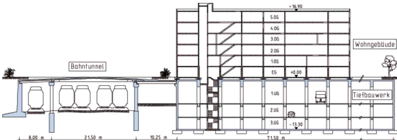
Bild 2. Regelquerschnitt des Tiefbauwerks mit Wohngebäuden und Bahntunnel Fig. 2. Typical sectional view of underground structure, apartment buildings and railway tunnel
