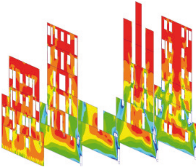
Bild 6. Vergleichsspannungen der Schotwände (Längswände und Decken ausgeblendet) Fig. 6. Equivalent stresses of high beams (longitudinal walls and slabs hidden)
