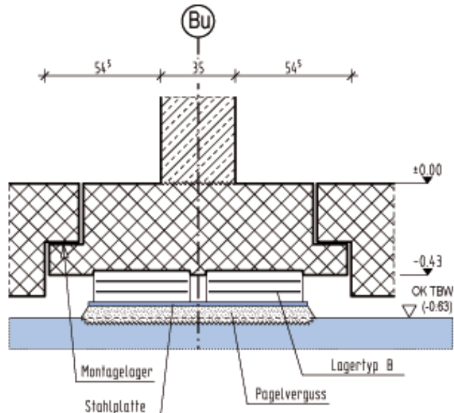
Bild 8. Geometrie Lagersockel Fig. 8. Dimensions of bearing
