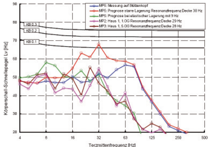
Bild 11. Verlauf der Schwingungsgeschwindigkeit Fig. 11. Characteristics of vibration speed
